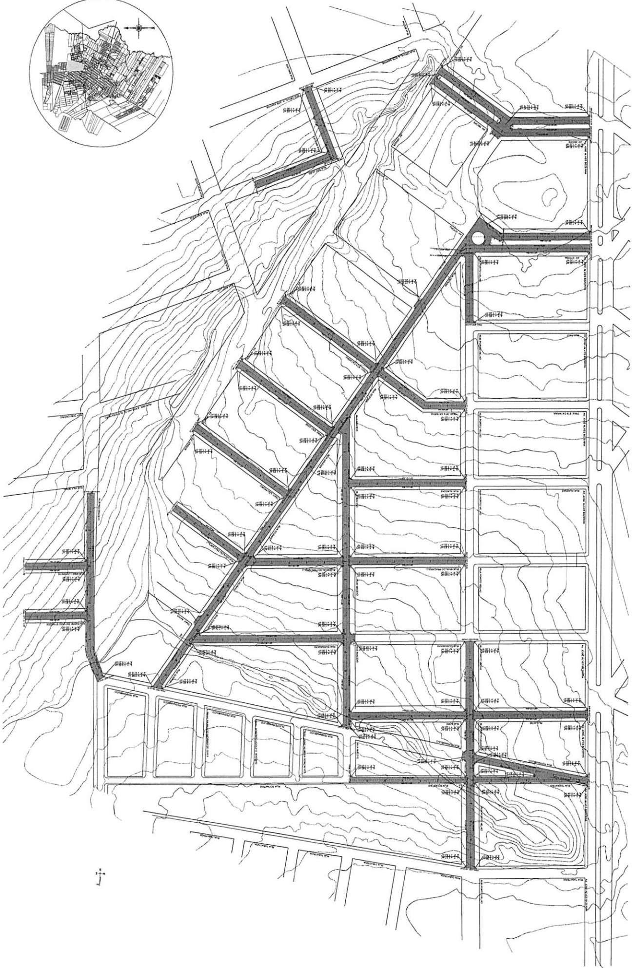
PLANTA GEOMÉTRICA PAVIMENTAÇÃO E EMBECADOURAS
